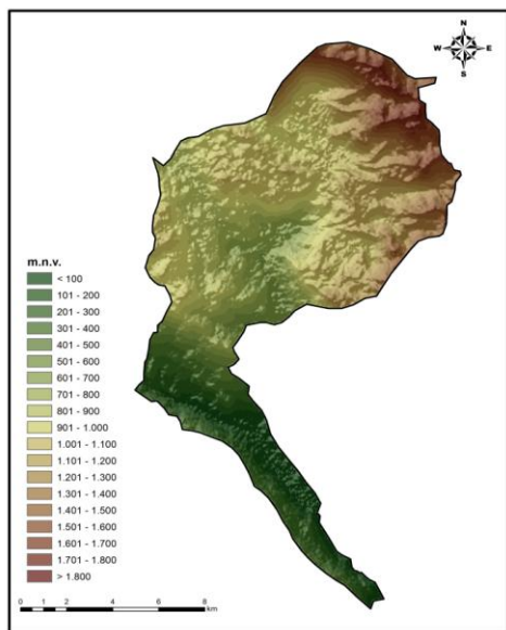
Sl. 7. Morfometrijska visinska raščlanjenost Sutorine
