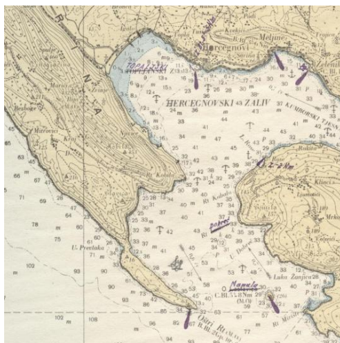
Sl. 10. Oceanografski pokazatelji u zalivu Herceg Novi
