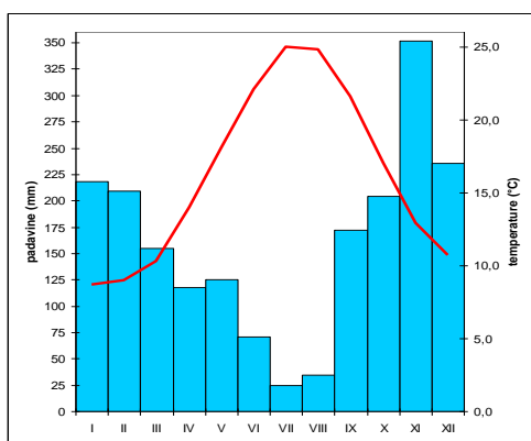
Sl. 11. Klima dijagram padavina (plavi stupci) i temperatura (crveni linijski grafikon)
