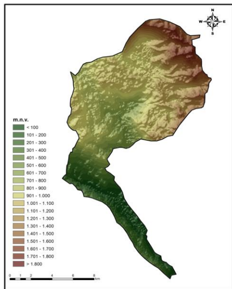
Sl. 7. Morfometrijska visinska raščlanjenost Sutorine
