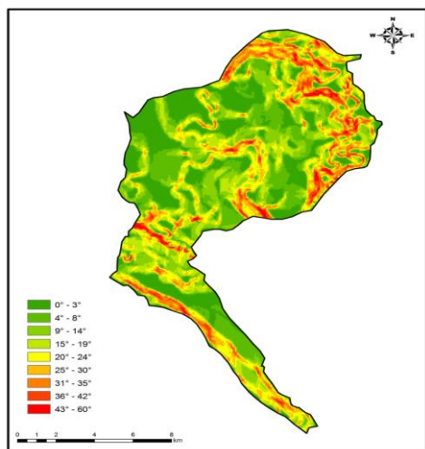
Sl. 9. Reljefna struktura Sutorine izražena nagibima
